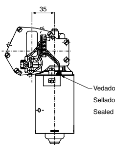
A Ângulo do flanco do dente: 90° - Nº de dentes: 42 - Passo: 0,68 Ángulo del flanco del diente 90° - Nº de dientes: 42 - Paso: 0,68 Tooth flank angle 90° - Number of teeth: 42 - Span: 0,68
